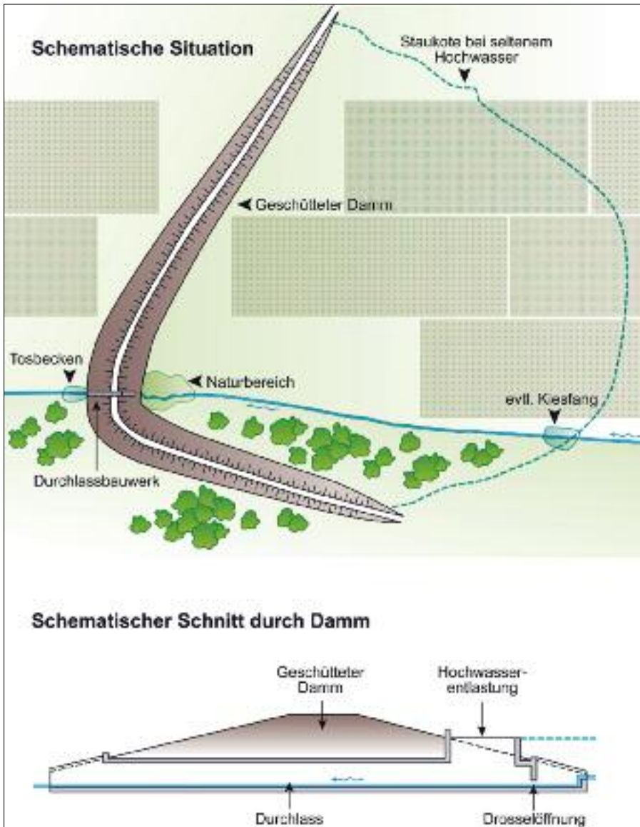
Ein typisches Hochwasserrückhaltebecken: Situation und Schnitt.
